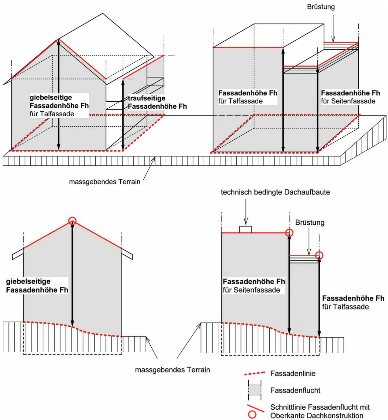
Figur 5.2 Fassadenhöhe
